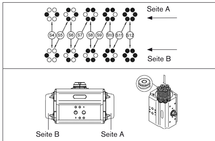
Bild 16: Deckelmontage
