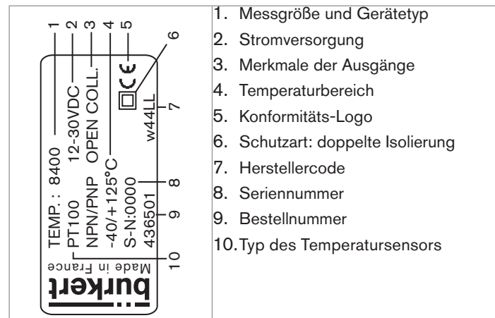
Bild 1: Typenschild des Geräts 8400 (Beispiel)
