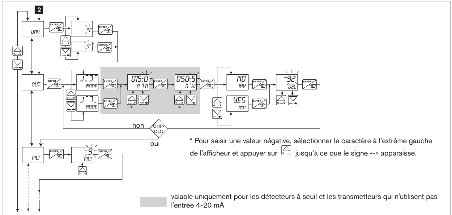
Fig. 24 : Déplacement dans le mode Calibration
