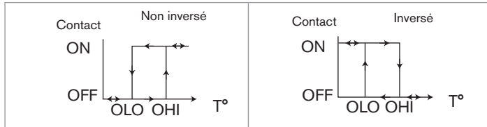
Fig. 26 : Changelement de la sortie en mode hystérésis
