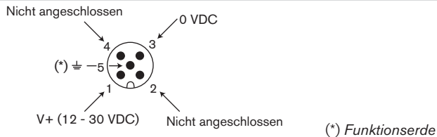
Bild 14: Belegung des 5-poligen M12-Gerätesteckers bei einer Version mit Relaisausgang
