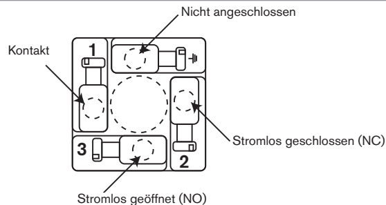
Bild 15: Belegung des Gerätesteckers nach EN 175301-803 (Anschluss des Relaisausgangs)
