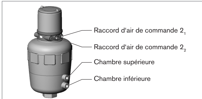
Fig. 10 : Raccordement pneumatique à l'actionneur
