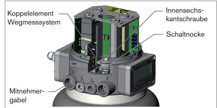
Bild 2: Koppelung Wegmesssystem
