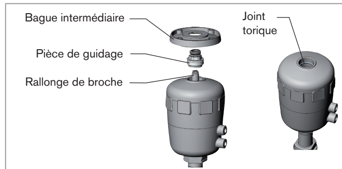
Fig. 5 : Démontez le kit d'adaptation 8630
