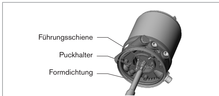
Bild 8: Ausrichten Puckhalter
