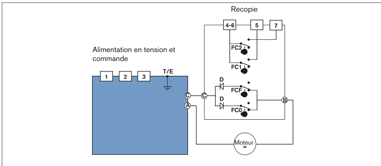
Figure 19 : Câblage interne de l'actionneur électrique
