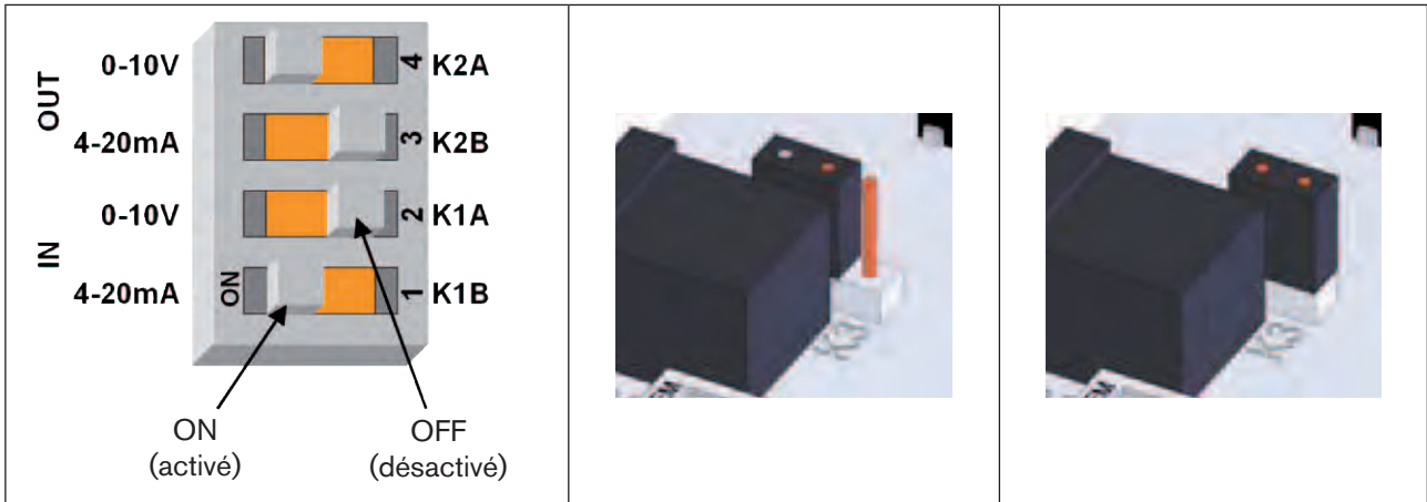
Figure 23 : Cavaliers K1 / K2
