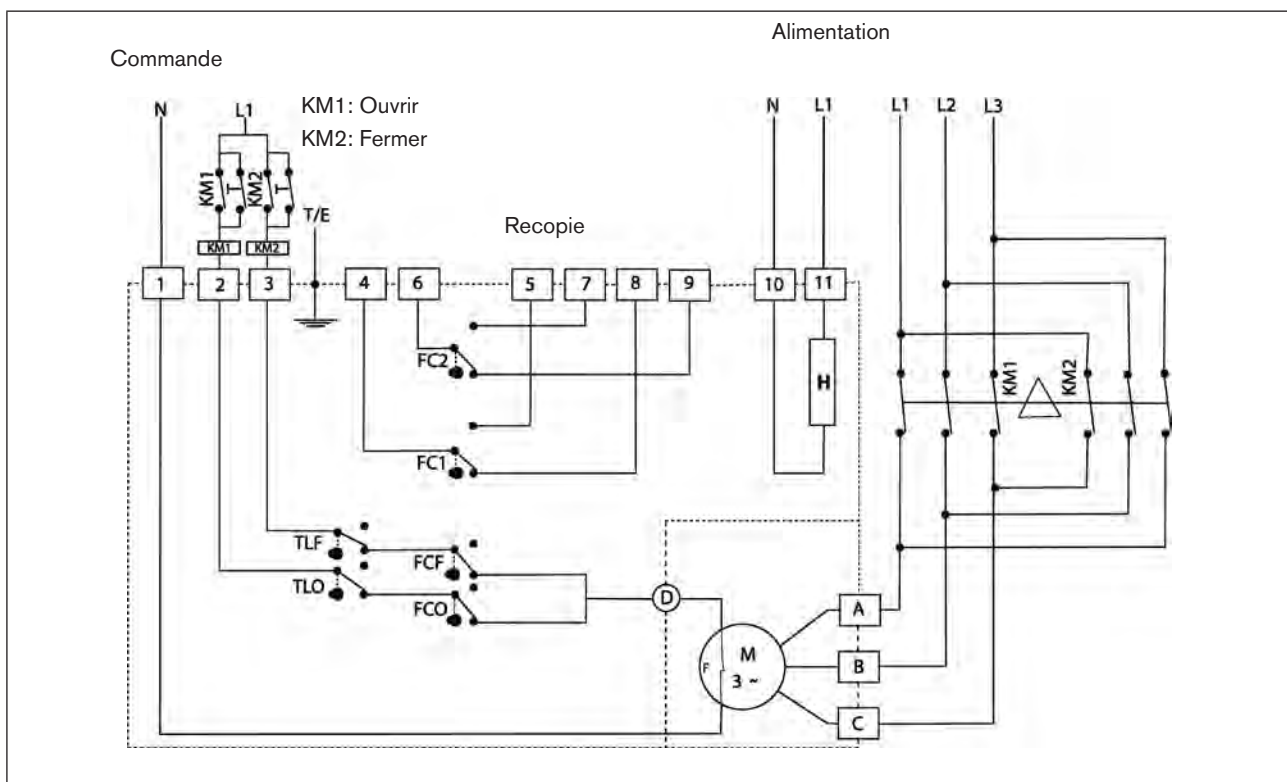
Figure 21 : Schéma électrique version 400 V courant triphasé
