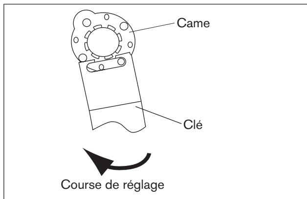
Figure 12 : Réglage des contacts de recopie dans le sens des aiguilles d'une montre
