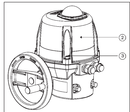
Bild 11: Haube Demontage
