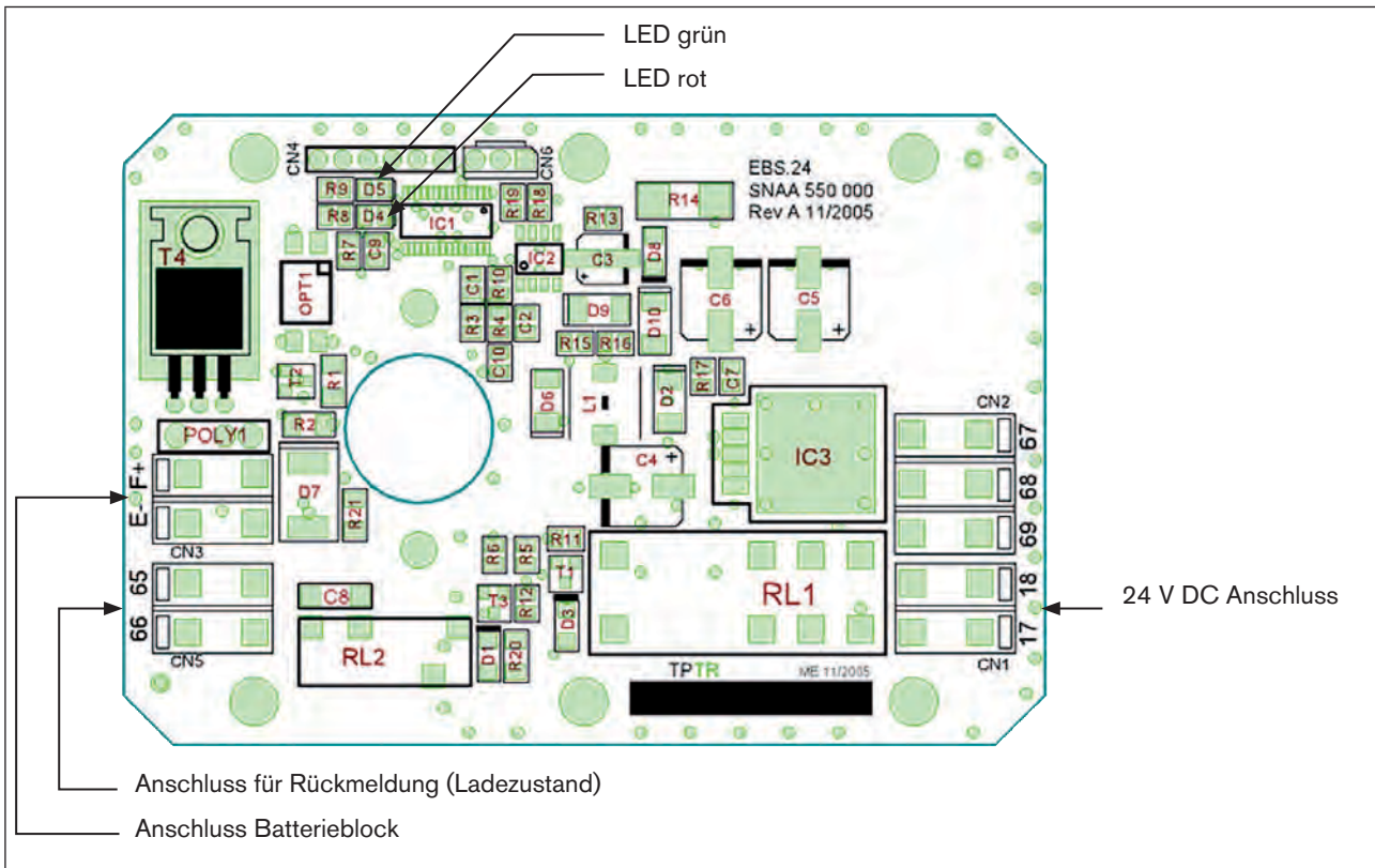
Bild 28: Darstellung: Elektronische Karte
